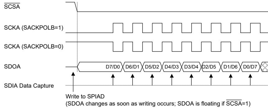
SPIA 从机模式时序图 – SACKEG=0
