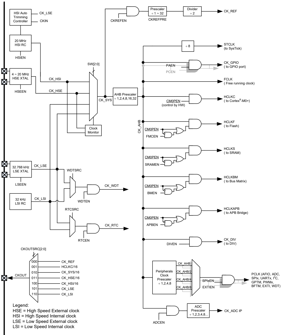
图 3. 时钟结构图
