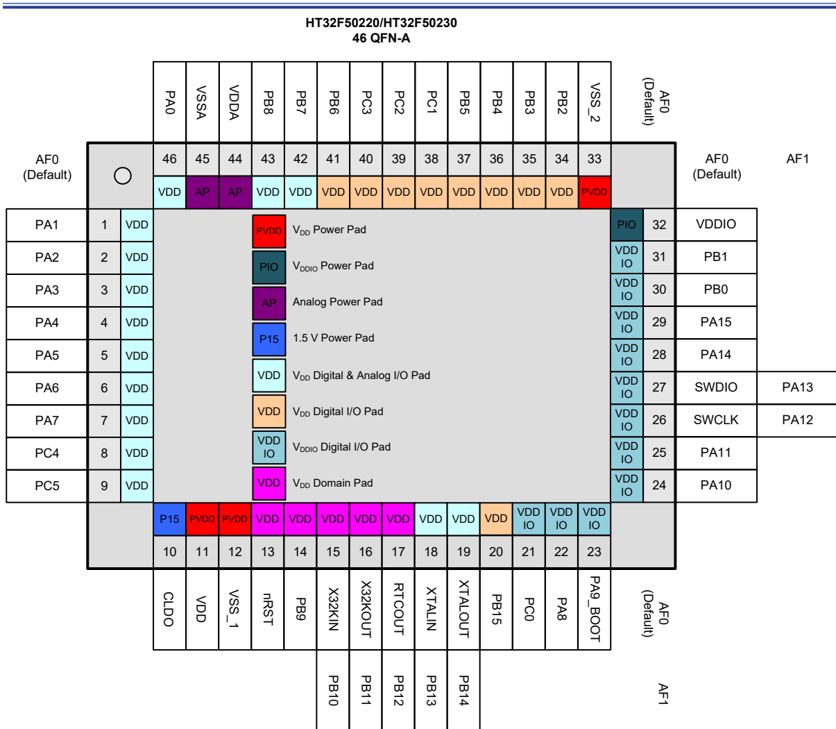
图 9. 46-pin QFN 引脚图
