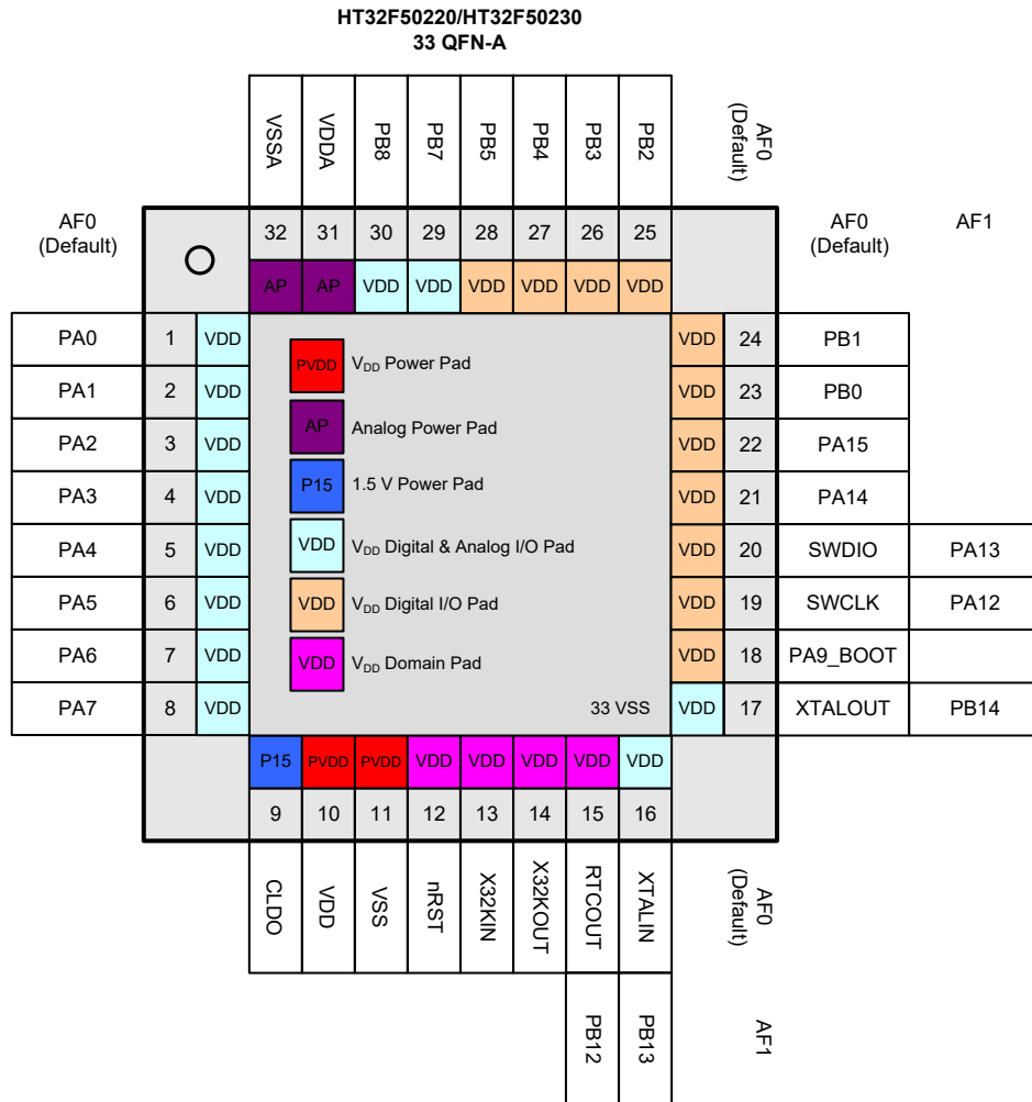
图 8. 33-pin QFN 引脚图
