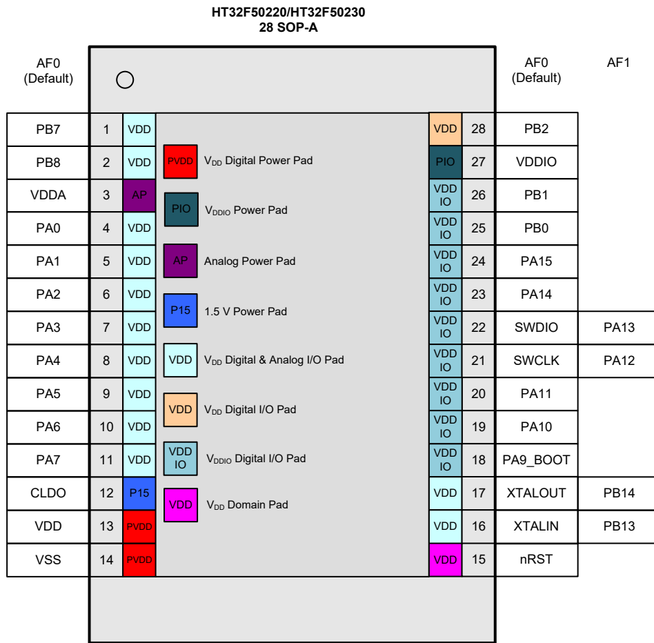
图 6. 28-pin SOP 引脚图
