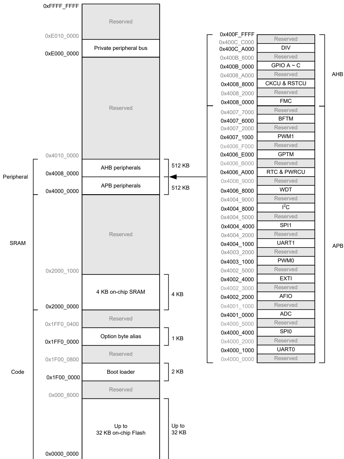
图 2. 存储器映射
