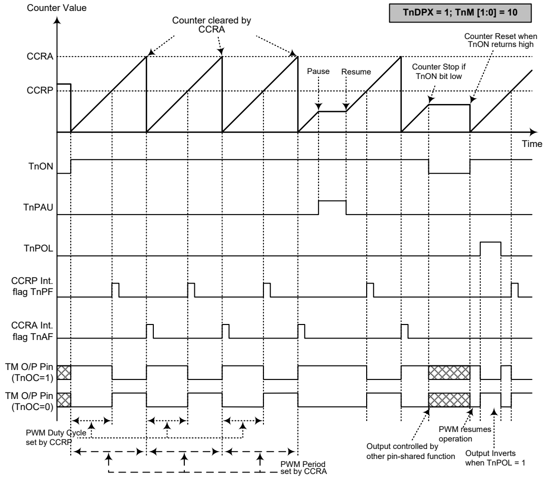
PWM 输出模式 – TnDPX=1 (n=2)
