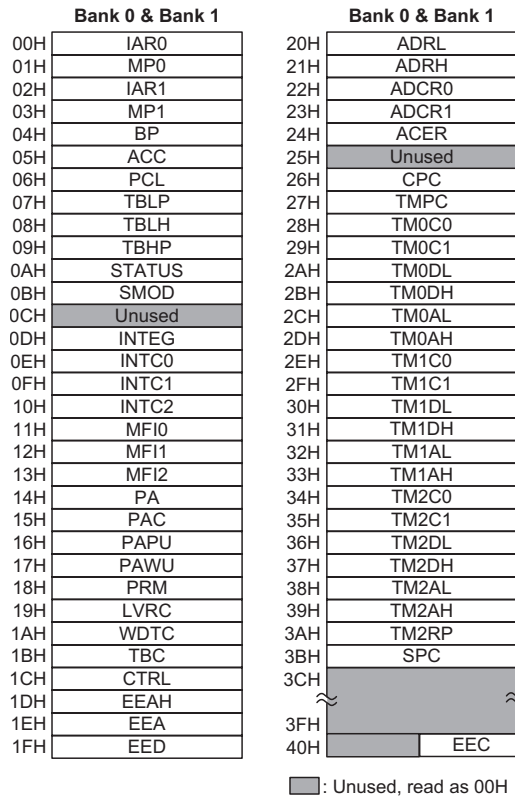
特殊功能数据存储器结构
