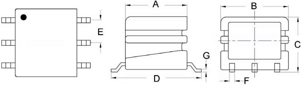
产品尺寸
