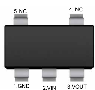
SOT-23-5
