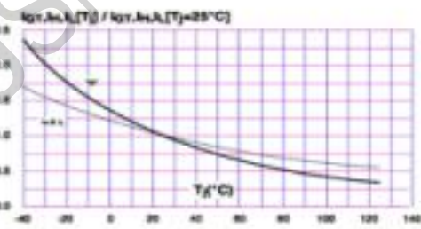
7、门级触发特性曲线
