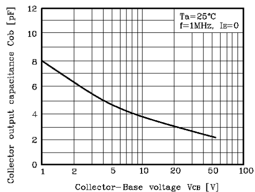
Fig. 5 C_{ob} - V_{CB}
