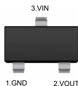
SOT-23-3
