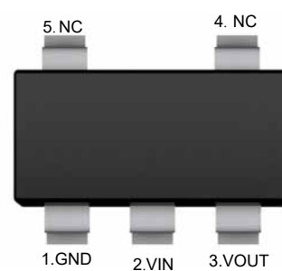
SOT-23-5
