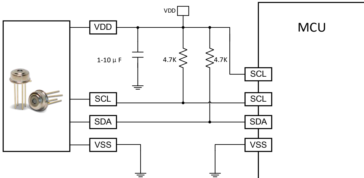
图9: 推荐电路
