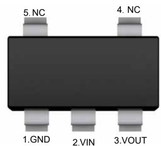
SOT-23-5
