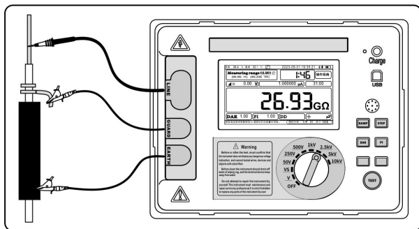
图 17（超高阻值三线测量接线方式）
