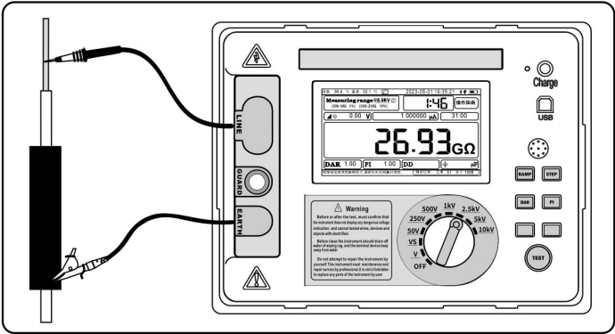
图 16（接常规两线测量接线方式）
