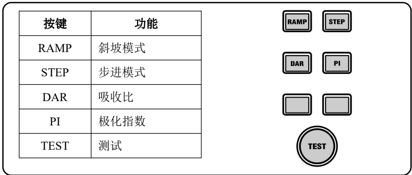
图 3 （按键图）
