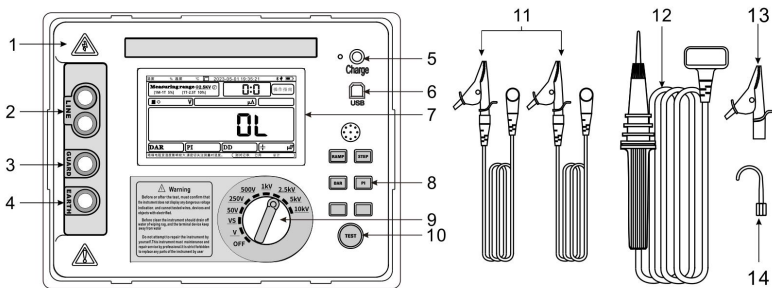
图 1 （仪表结构图）
