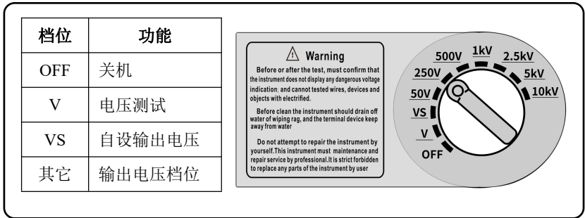
图 2 （旋钮档位图）
