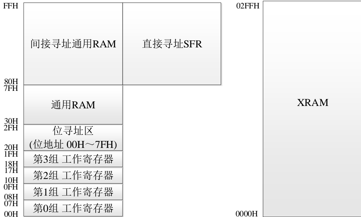
Figure 3-2 数据存储器示意图
