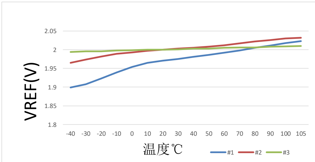
Figure 21-4 内部参考电压 2V - 温度特性曲线图
