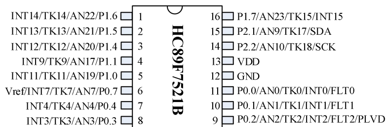
Figure 1-3 SOP16 引脚配置图
