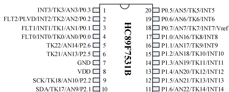
Figure 1-2 SOP20 引脚配置图
