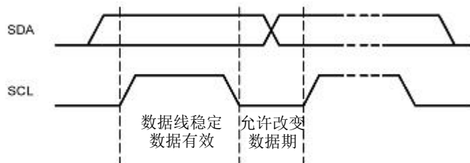
Figure 15-3 IIC 总线上数据的有效性
