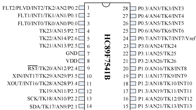
Figure 1-1 SOP28 引脚配置图
