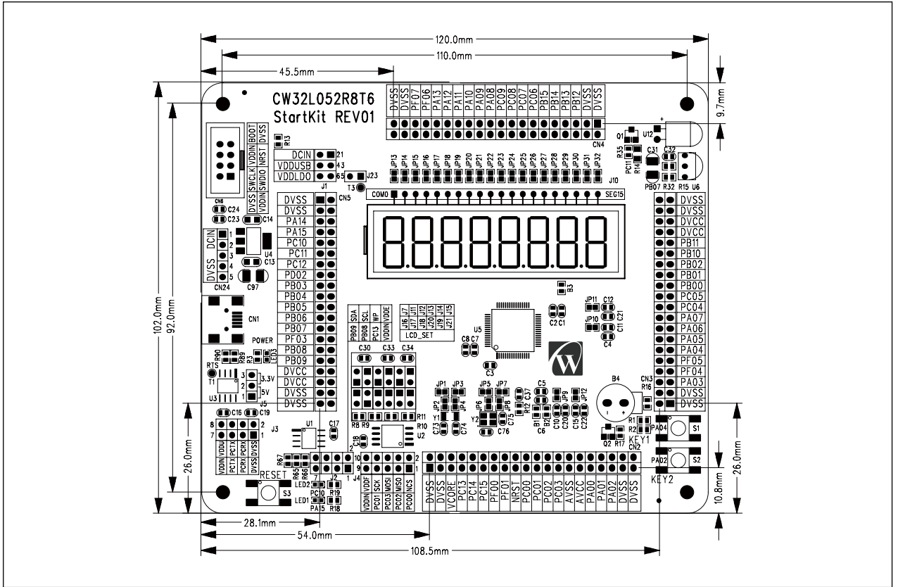
图 6-2 机械尺寸
