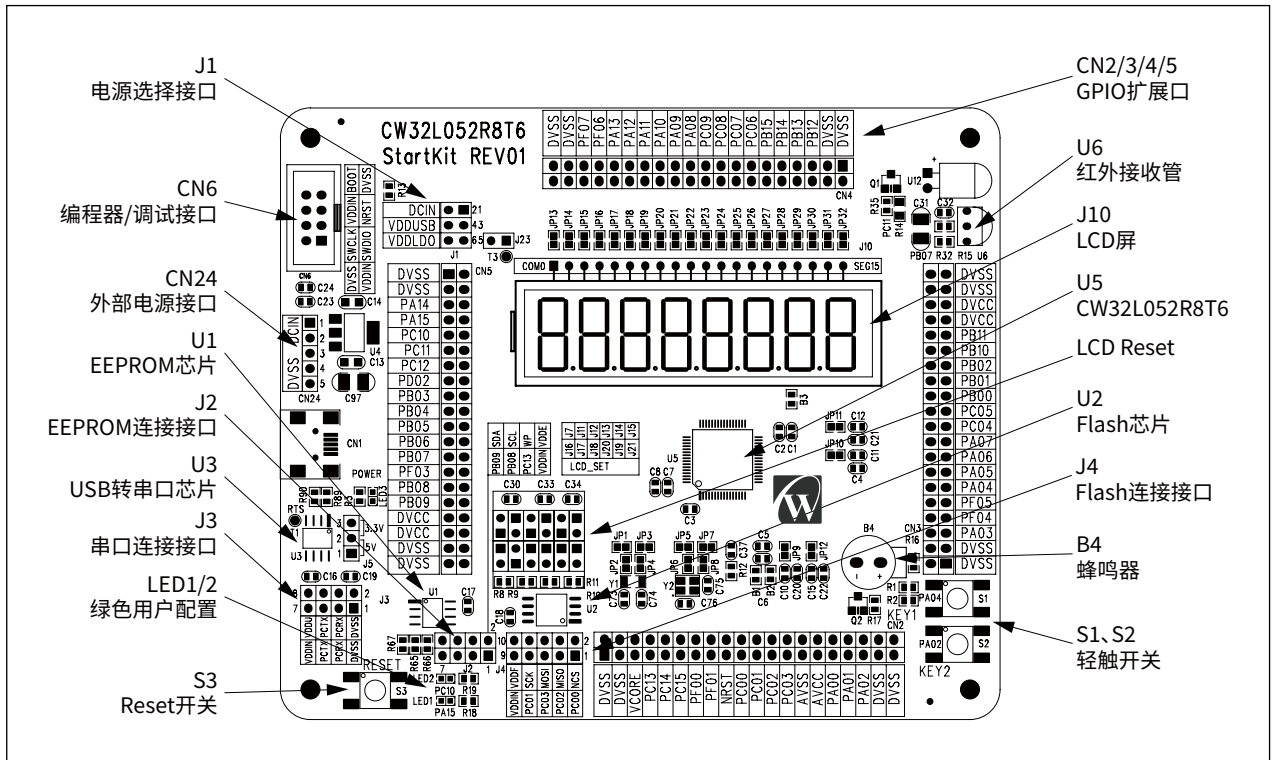
图 6-1 顶层器件布局
