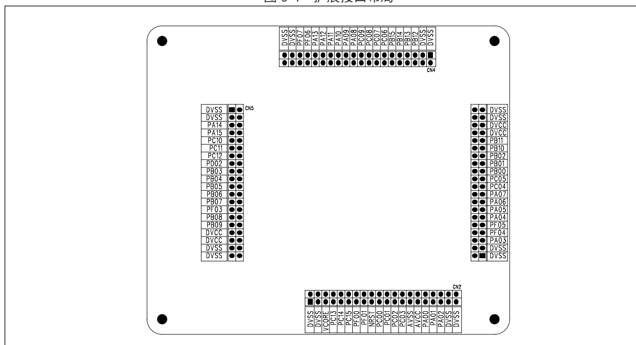
图 6-4 扩展接口布局
