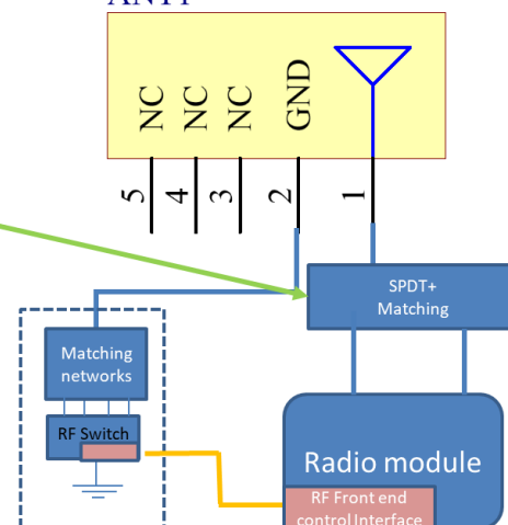
TAOGLAS_PCS.50.A ANT1
