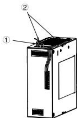
① 端子接上连接线后, 铺设和对齐 连接线; ② 通过外壳两侧的缺口, 用电线捆 扎条, 固定连接线。
