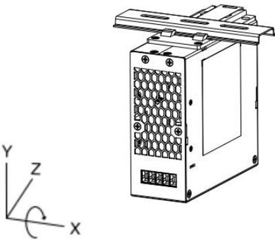
旋转安装位置(270° X-轴)
