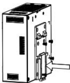
① 安装通用DIN导轨适配器 (侧面正装, 需撕标签纸)
