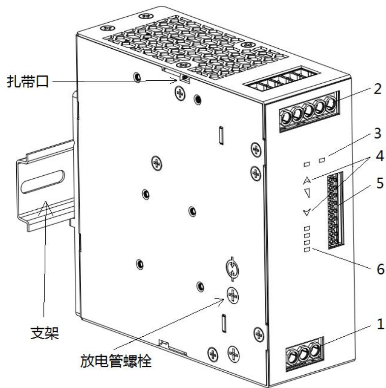
图 1：LIHF240-23Bxx 外观信息
