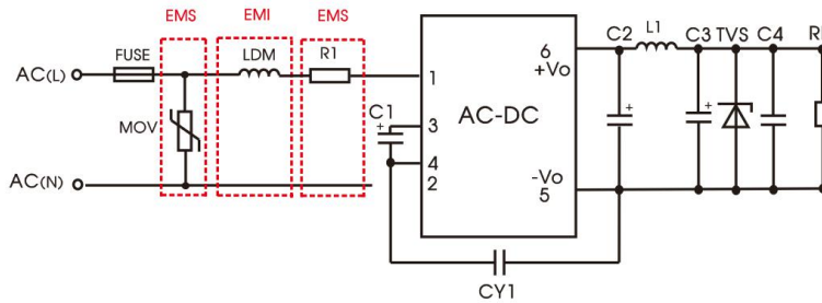
推荐电路 4
