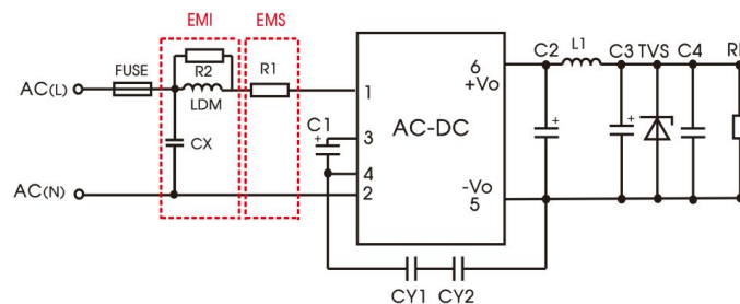
推荐电路 2
