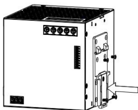
① 安装通用DIN导轨适配器 (侧面正装，需撕标签纸)
