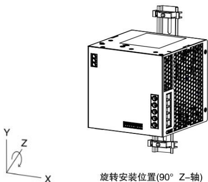
旋转安装位置(90° Z-轴)
