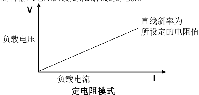
图3-3 CR模式电压电流关系图
