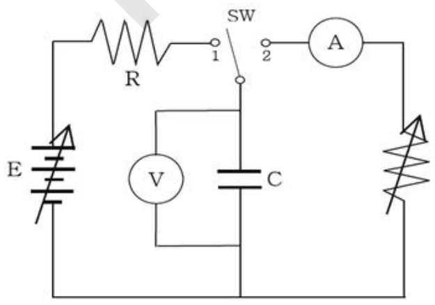
图1 容量测试电路图
