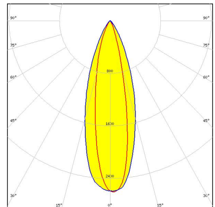
FP18682_LISA3CSP-O2-90-CLIP16
