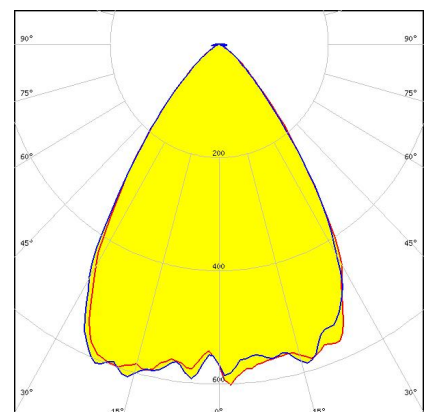
FP16611_LISA3CSP-WWW-PIN
