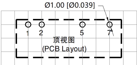
注：栅格距离为 2.54*2.54mm
