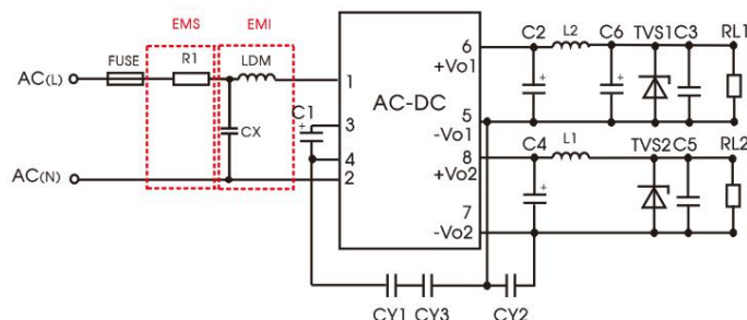
推荐电路 2
