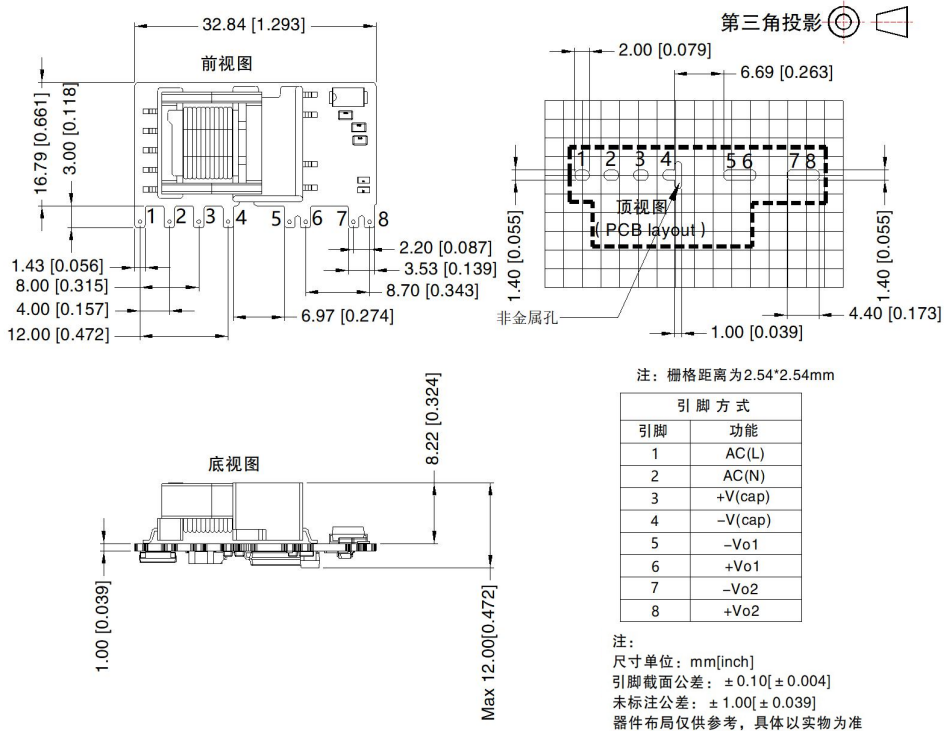
LS05-13Hxx 系列外观尺寸图
