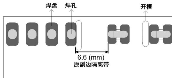
LS05-13Hxx 系列推荐焊盘
