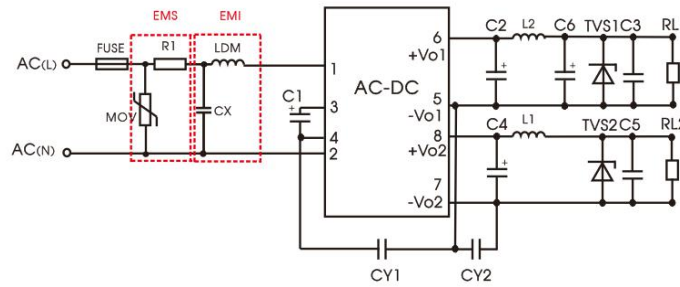
推荐电路 3
