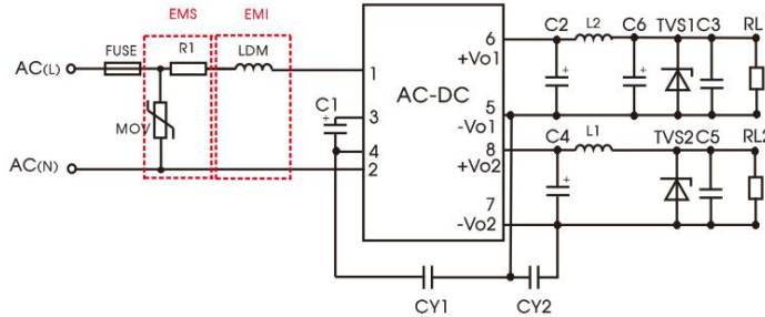
推荐电路 4
