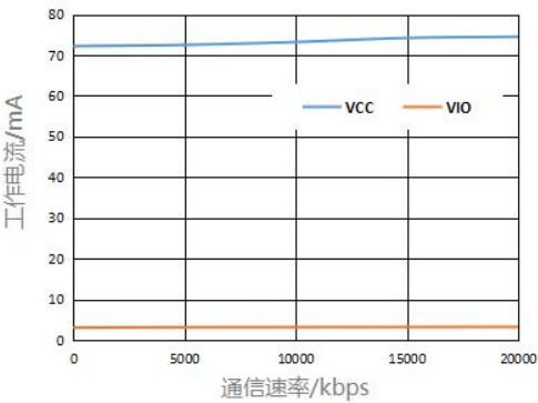
图 1.工作电流 vs. 通讯速率
