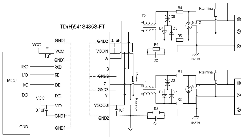
图 13.端口保护推荐电路
