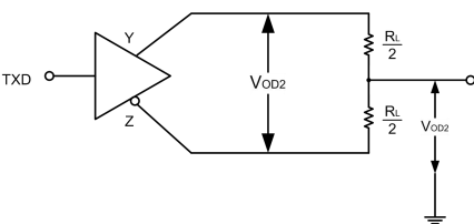
图 7.差分输出测试电路
