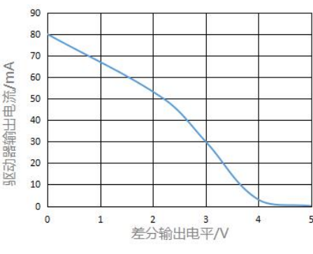
图 4.驱动器输出电流 vs. 差分输出电平
