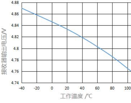
图 5.接收器输出高电平 vs. 工作温度
