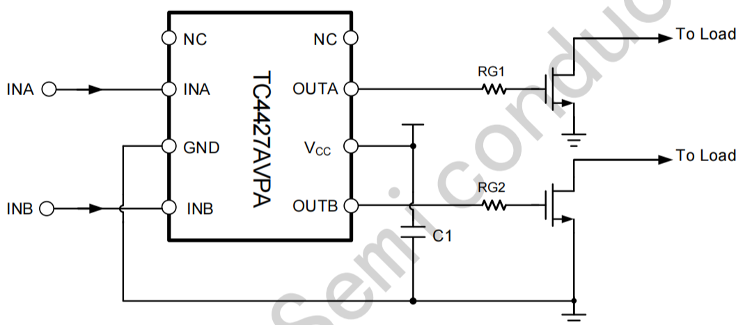
图 8-1 TC4427典型应用电路图
