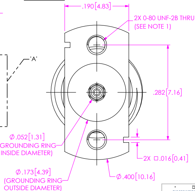
FIG 1 240-J-P-EP-ST-CM-X-X SHOWN
