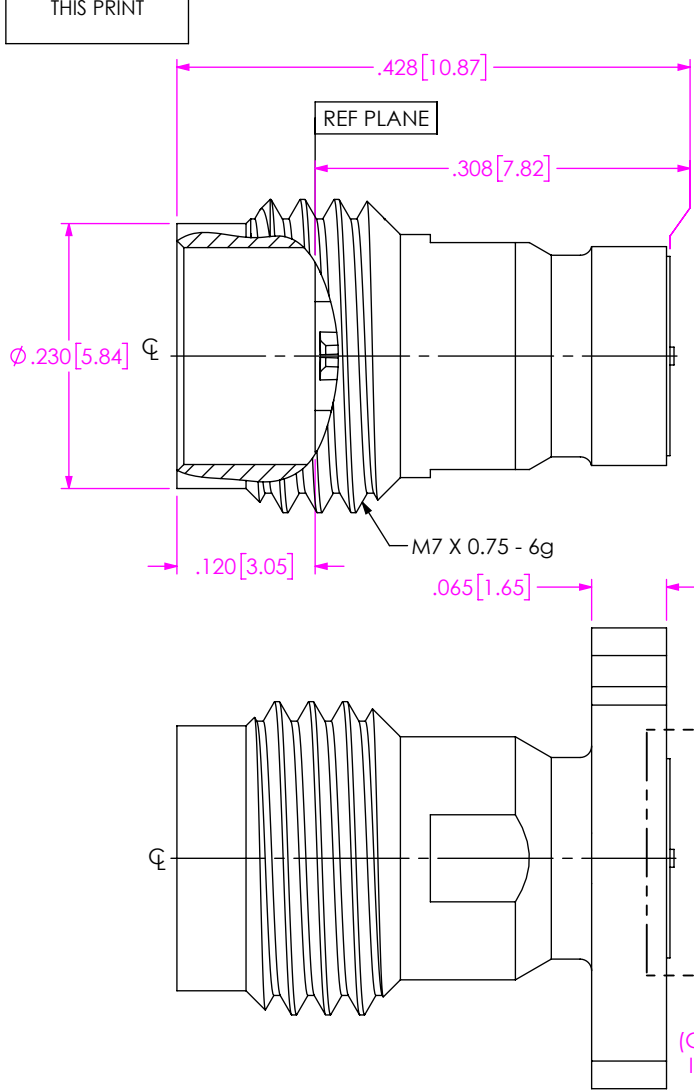
FIG 1 240-J-P-EP-ST-CM-X-X SHOWN
