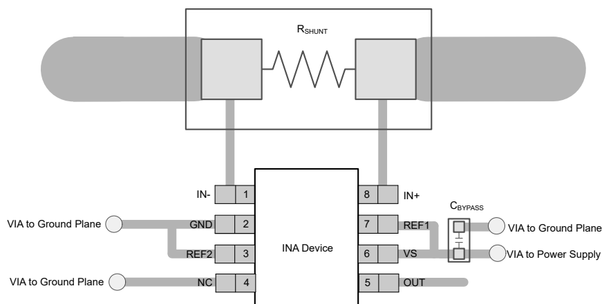
Figure 9-3. INA241x-Q1 SOT-23 (DDF), SOIC (D) and VSSOP (DGK) Package Recommended Layout
