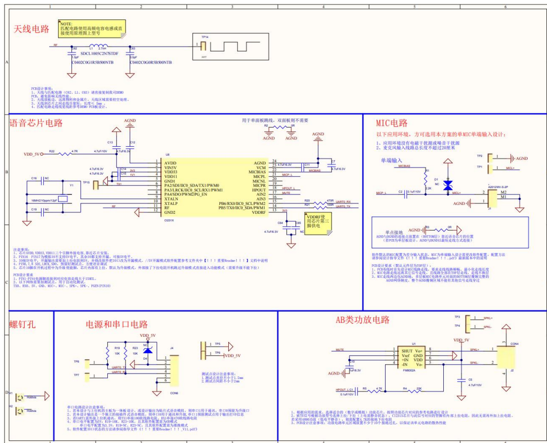
图 6-1 CI2312 方案的应用参考电路图
