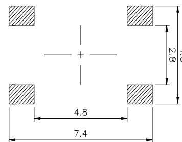
PCB. 焊接图
