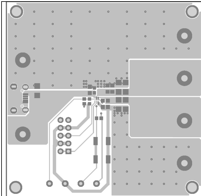
Figure1 Top Layer
