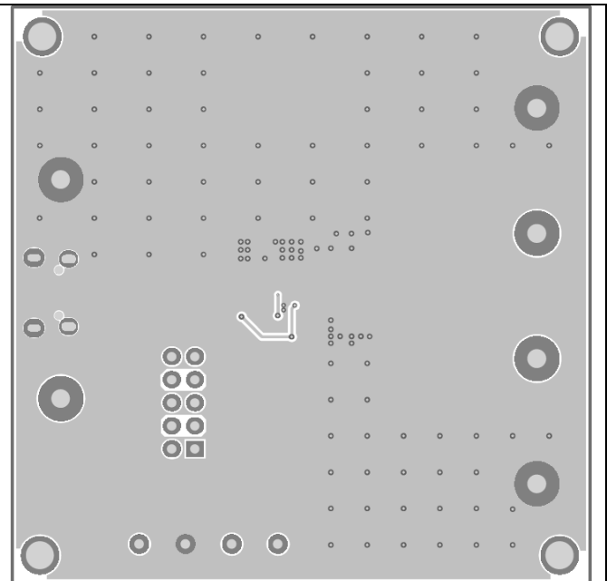
Figure2 Bottom Layer
