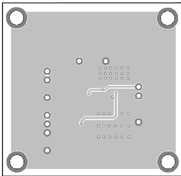
Figure 3—Bottom Layer
