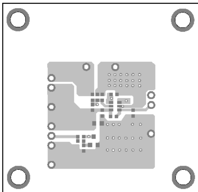
Figure 2—Top Layer
