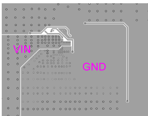
Bottom Layer
