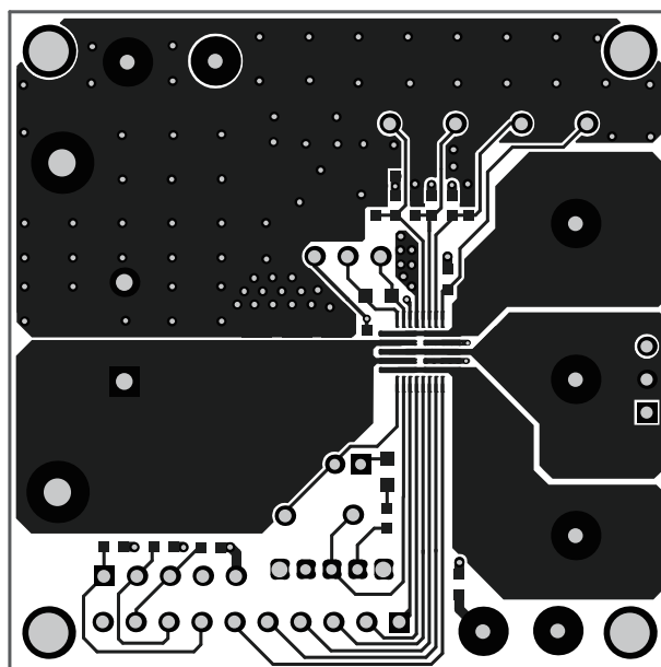
Figure 2—Top Layer
