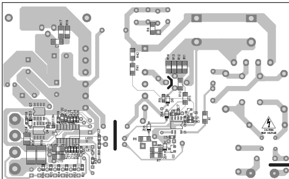
Figure 2—Bottom Layer
