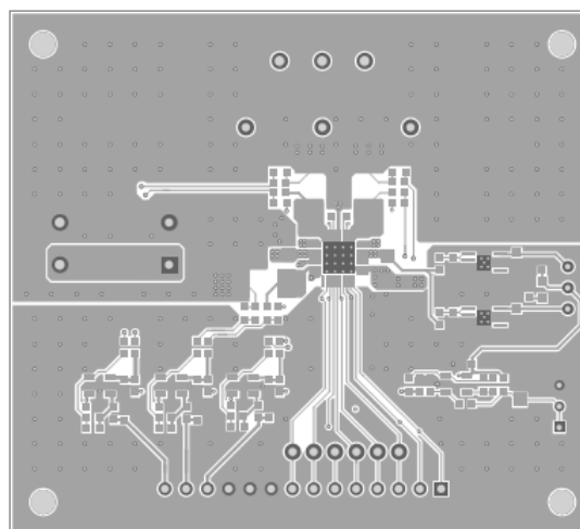
Figure 2—Top Layer
