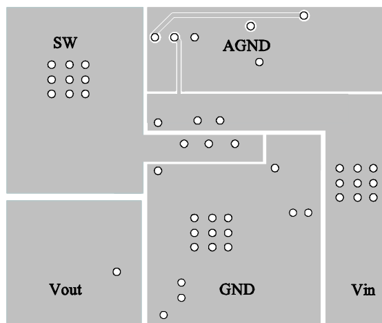
Bottom Layer
