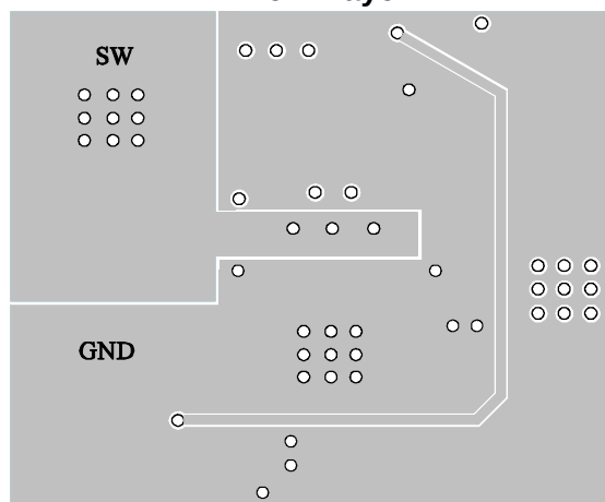
Inner2 Layer
