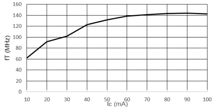
f_T vs I_C
