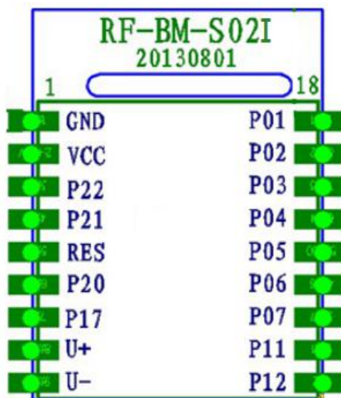
图 1 引脚定义
