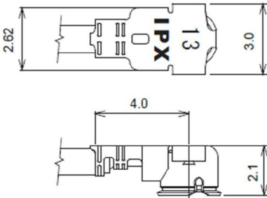
图 4 IPEX 线端规格
