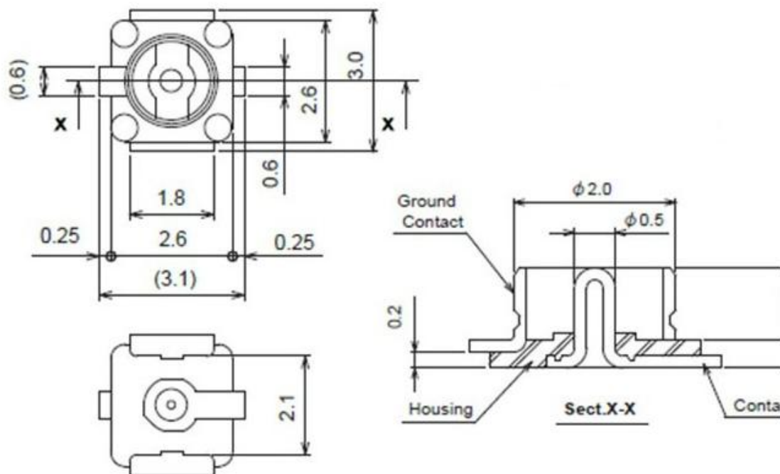
图 3 IPEX 板端规格
