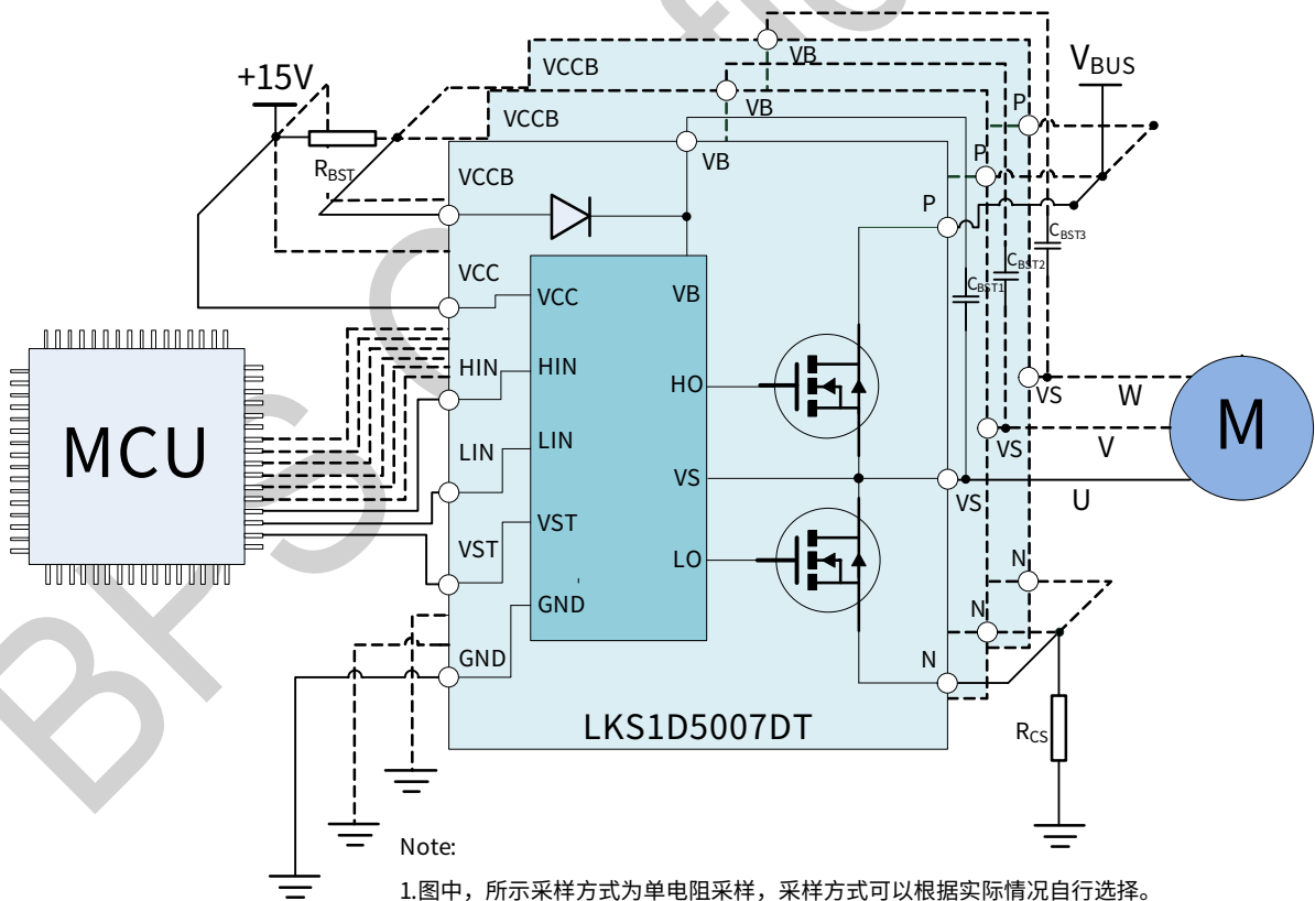
图 1. LKS1D5007DT 典型应用图
