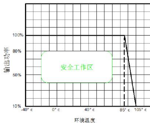
温度曲线图
