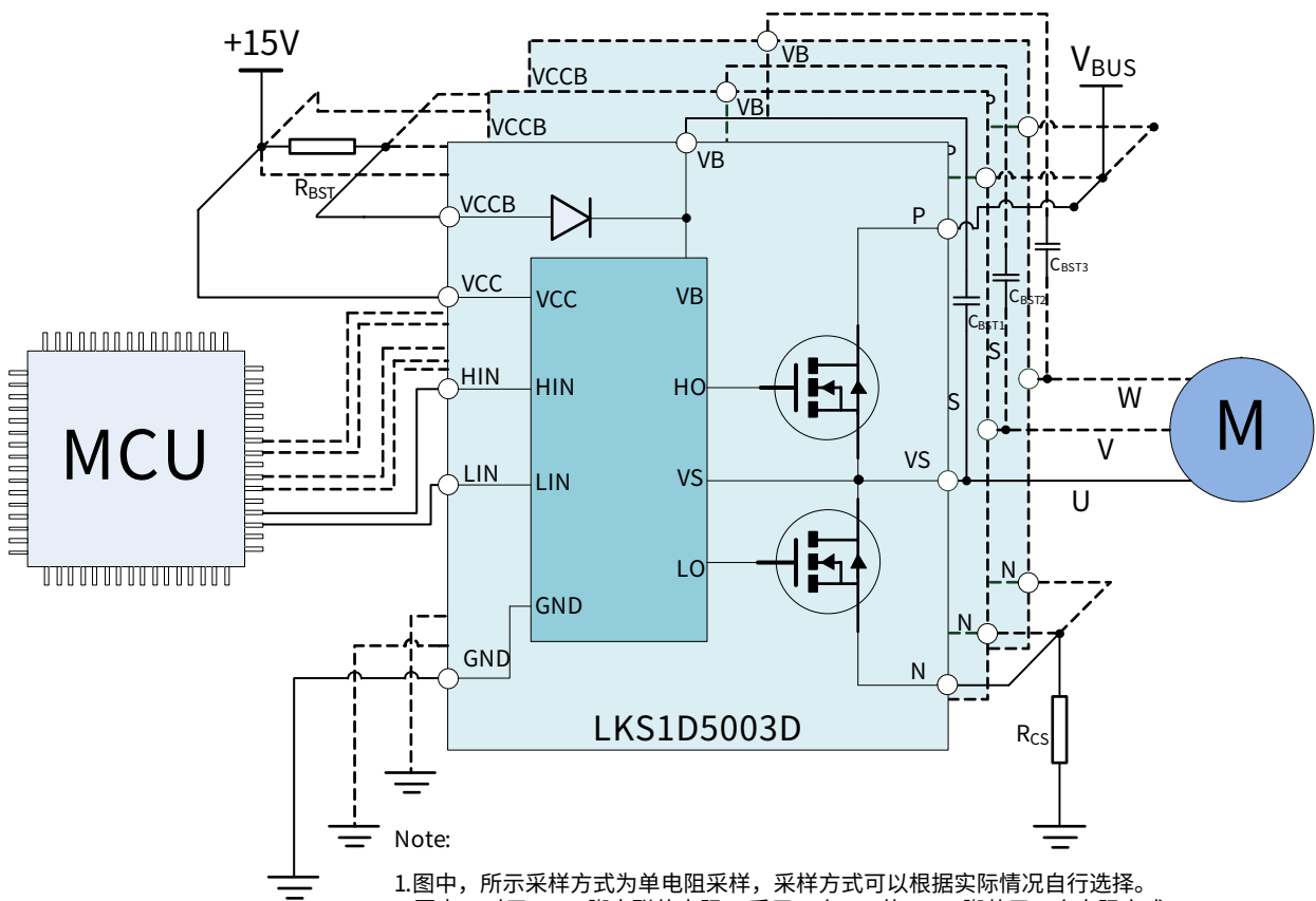
图 1. LKS1D5003D 典型应用图
