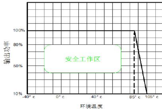
温度曲线图
