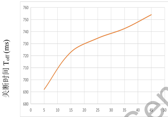
图.11 LED 关断时间-正向电流特性
