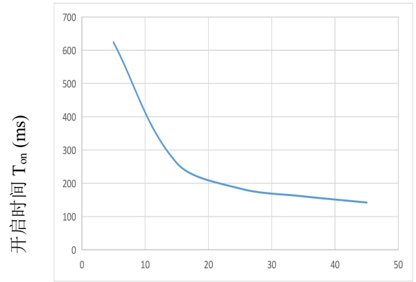
图.10 LED 开启时间-正向电流特性
