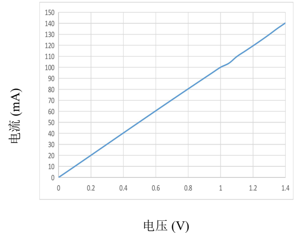
图.8 输出端电流-电压特性
