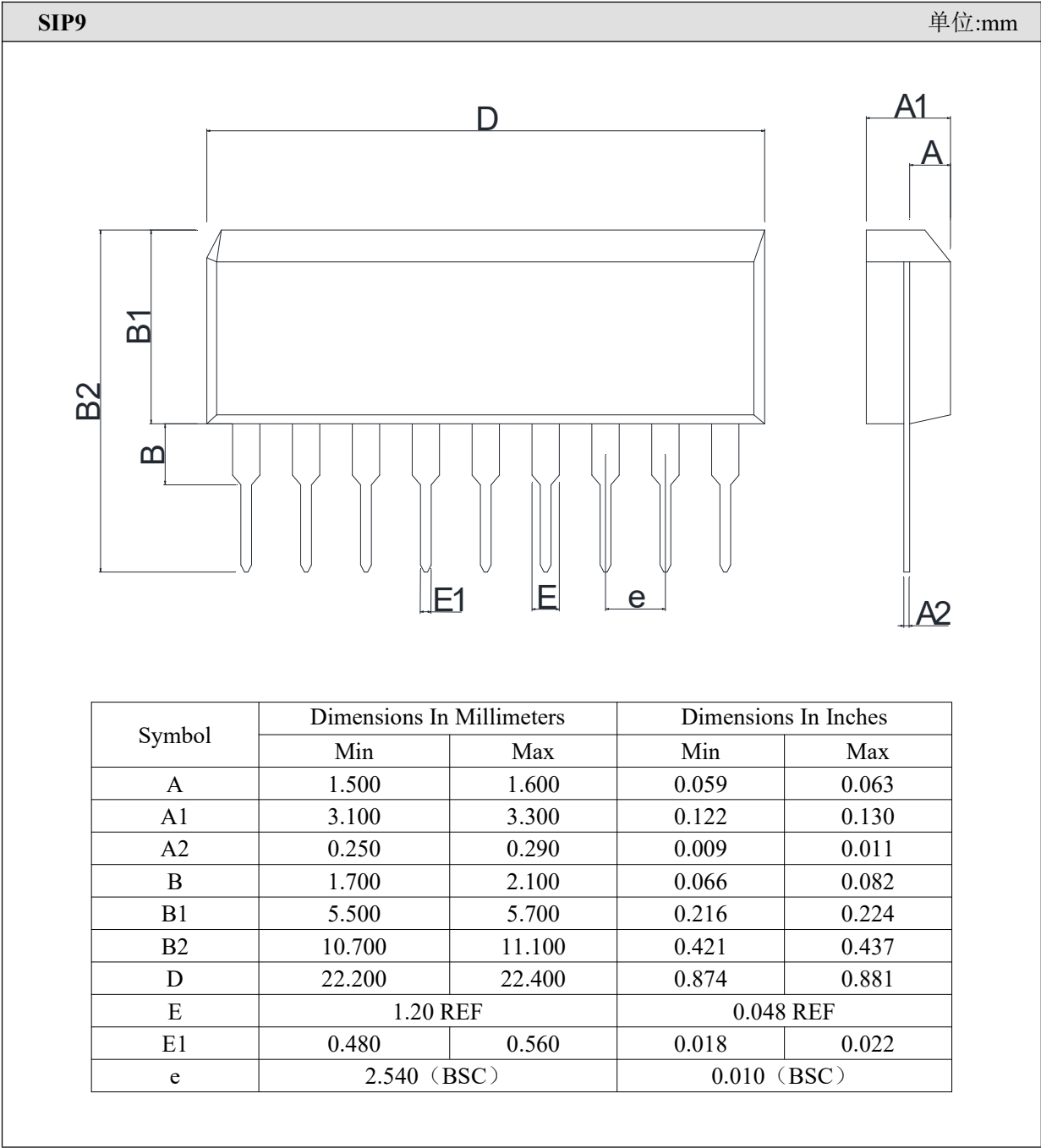
封装外形图:
