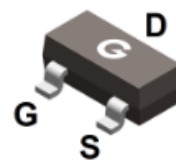
BL2300 SOT-23
