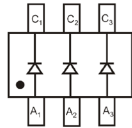
SOT-363
