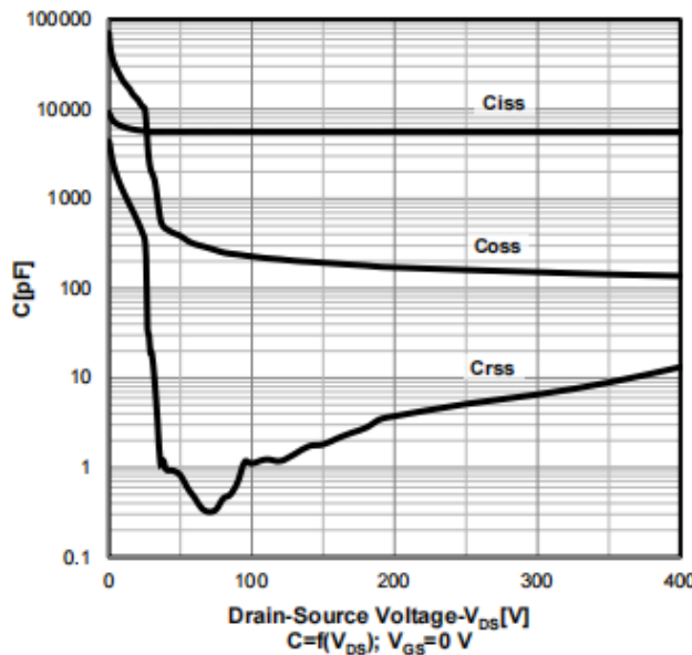
Typ. capacitances
