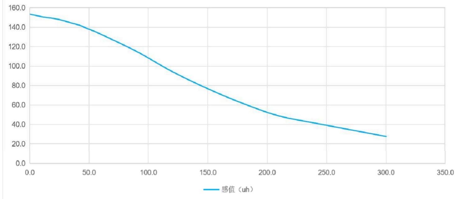
饱和电流曲线图
