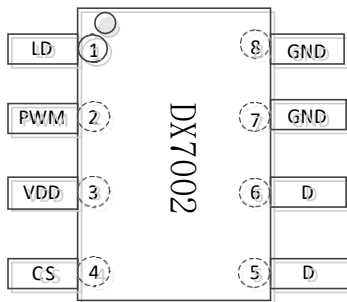
图 5.1 DX7002 管脚图
