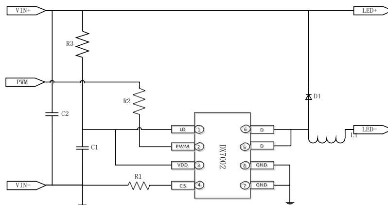
图 4.1 DX7002 应用电路
