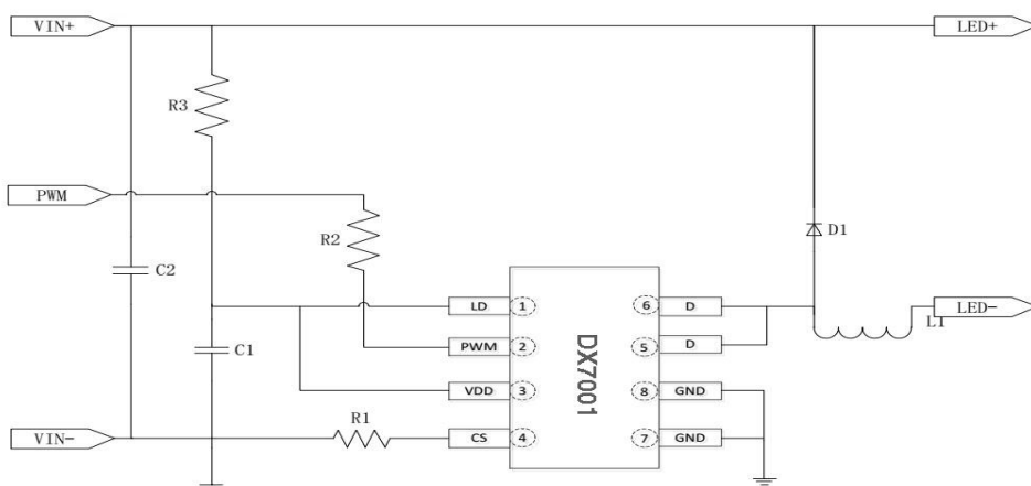
图 4.1 DX7001 应用电路
